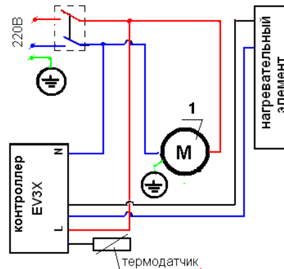
1 эп/дв. вентилятора нагревательного элемента
